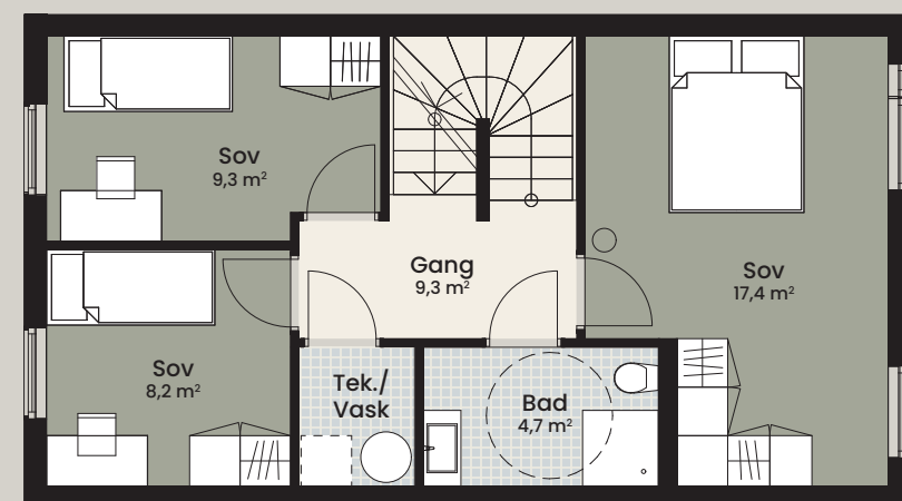
2. etasje
