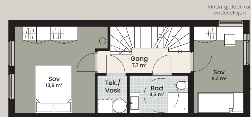
2. etasje
