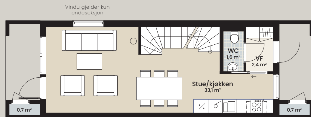
1. etasje
